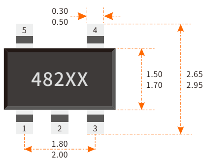
SOT-23-5L SO封装
