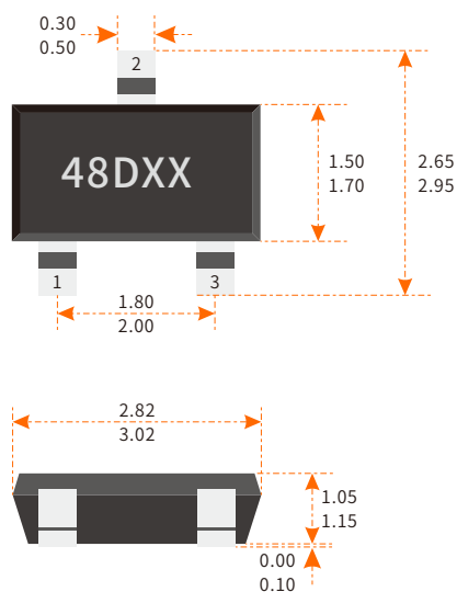
SOT-23 SO封装
