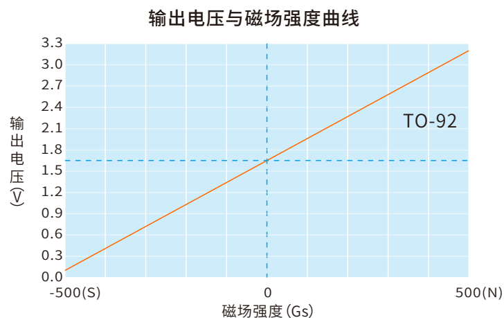
HAL9303R SOT-23示例图
