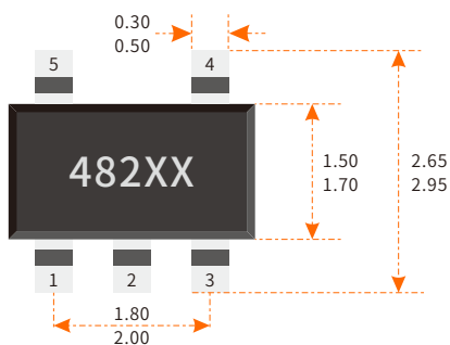
SOT-23-5L SN封装
